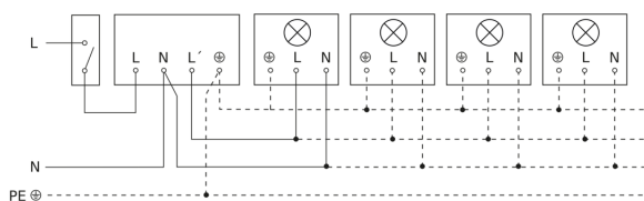
Schaltplan Leuchte ohne vorhandenen Nullleiter
